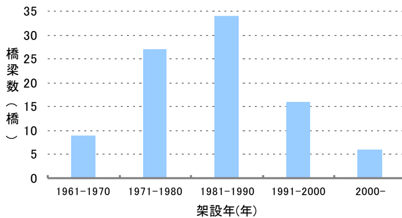
図 1 架設年別の橋梁数
