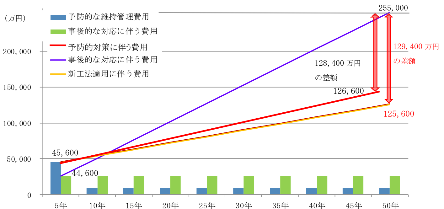
図 3 保全・更新費用の推移
