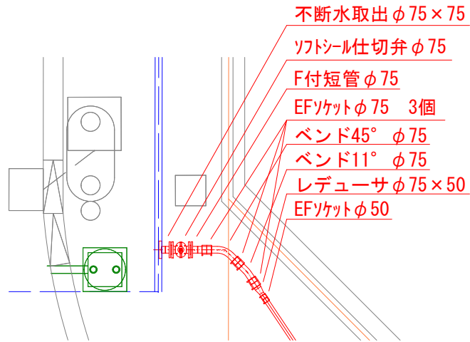
詳細(1) (箇所①起点部)
