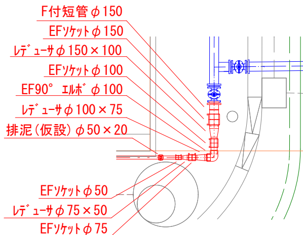
詳細(2) (箇所①終点部)
